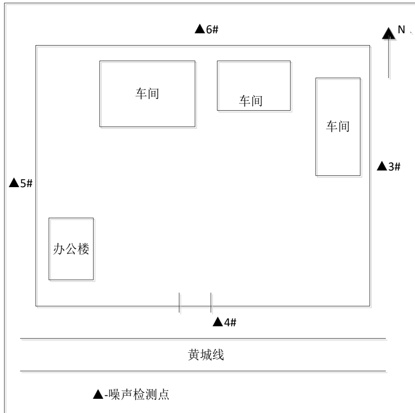
图 7-2 舟山神鹰车辆配件制造厂总平面布置图及厂界噪声布点示意图
